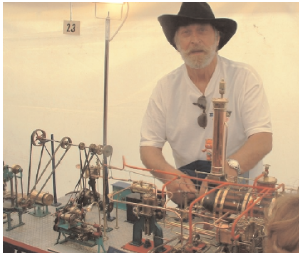
La maquette de la salle des machines du remorqueur Iroise, a été réalisée à l'échelle 1/40 ème par Gilbert Petitdemange
